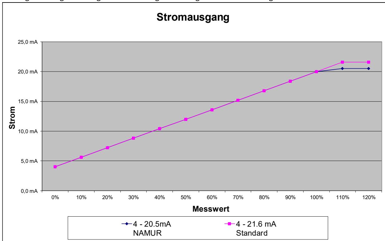
Diagramm 2: Stroma Ausgang als NAMUR oder Standard
