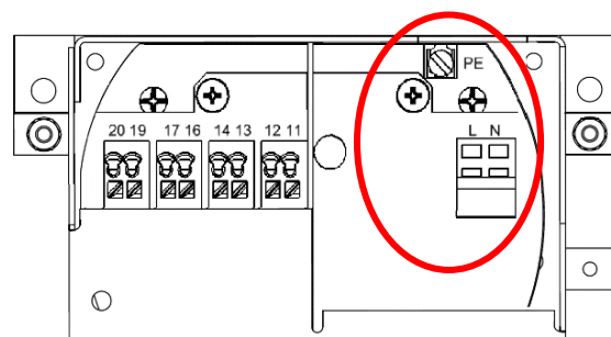
Netzanschlussklemmen UMC4-RM
